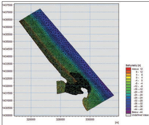
Hình 7. Lưới tính toán 2 chiều khu vực cửa Đà Nông
