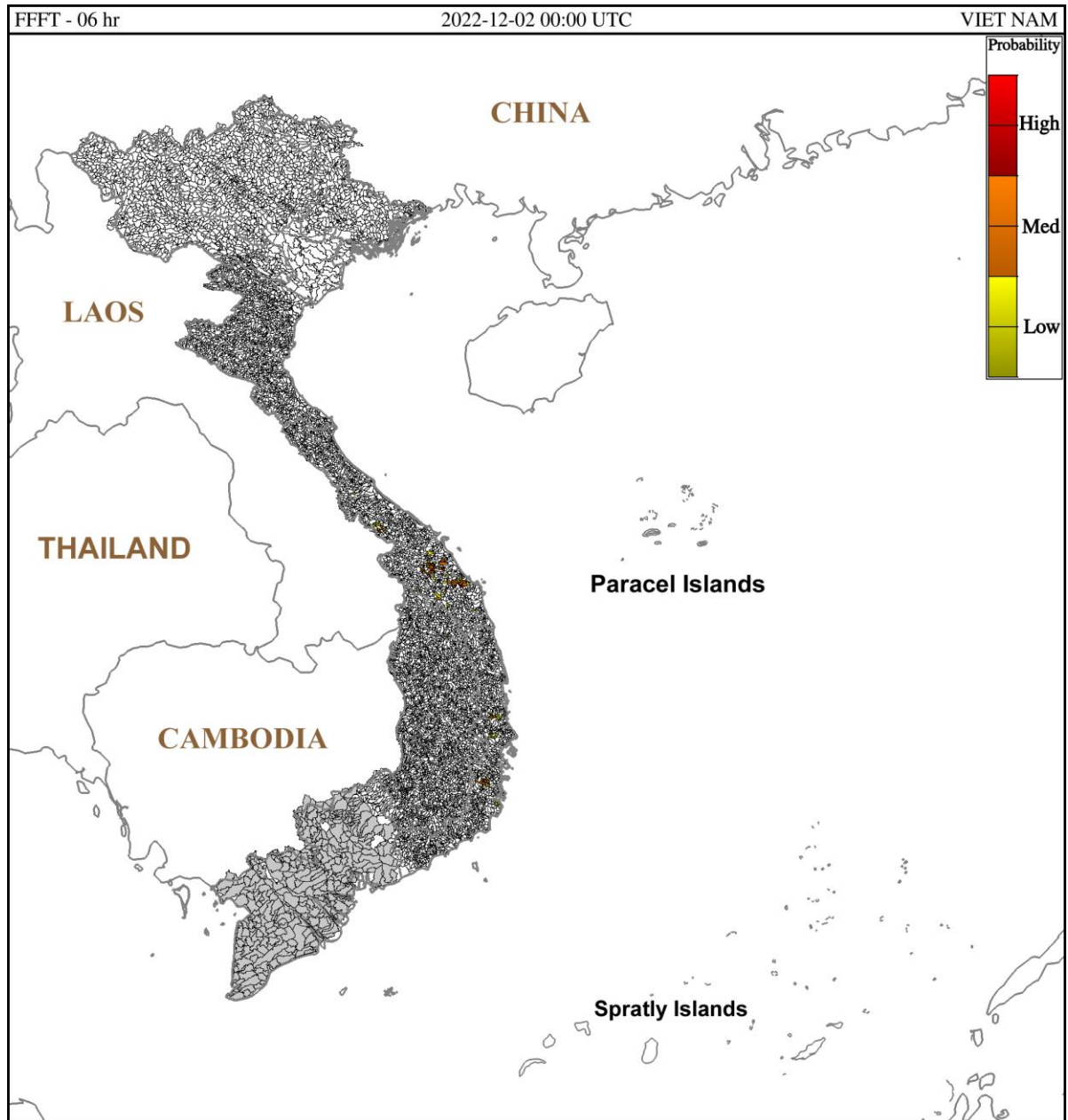
Hình 1. Nguy cơ lũ quét trong 6 giờ tới tại các lưu vực từ 07h ngày 02/12/2022 giờ địa phương
