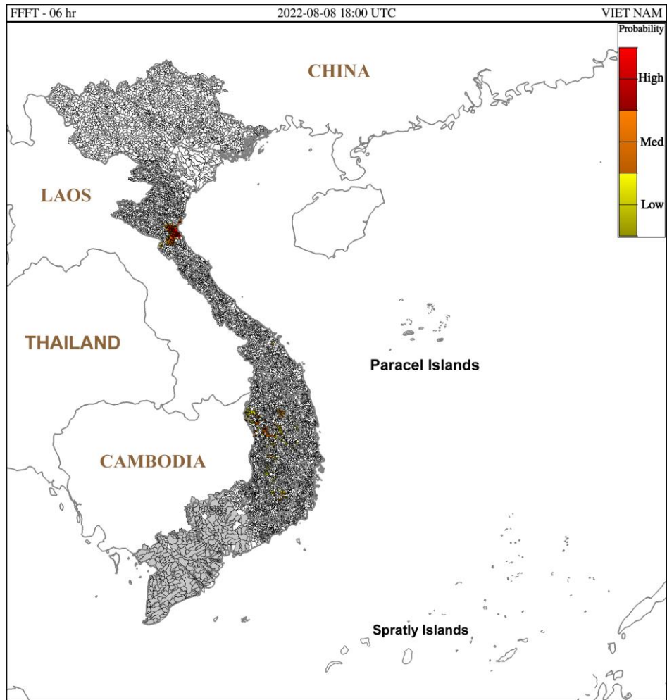
Hình 1. Nguy cơ lũ quét trong 6 giờ tới tại các lưu vực từ 01h ngày 09/08/2022 giờ địa phương
