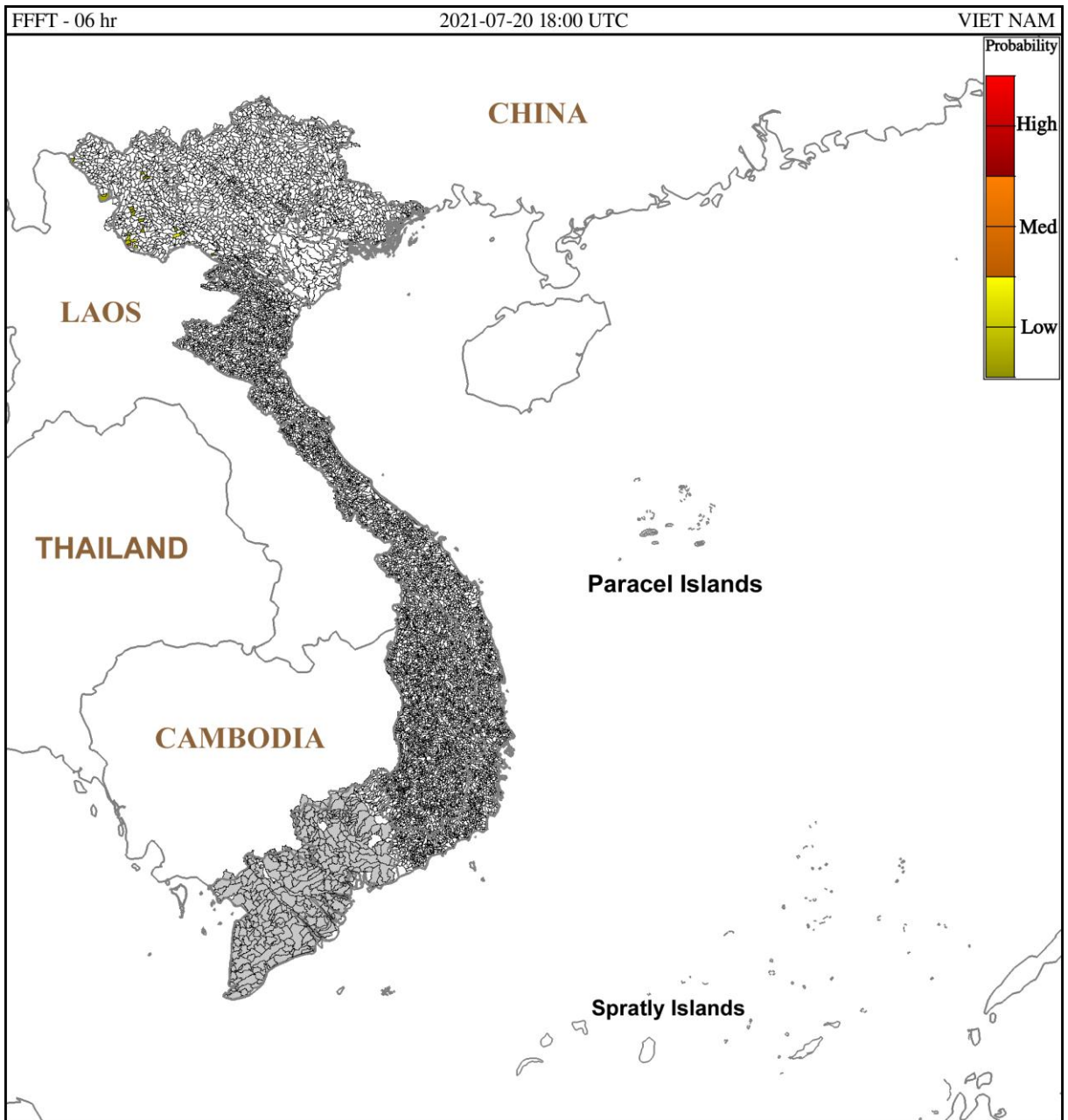
Hình 1. Nguy cơ lũ quét trong 6 giờ tới tại các lưu vực từ 01h ngày 21/07/2021 giờ địa phương
