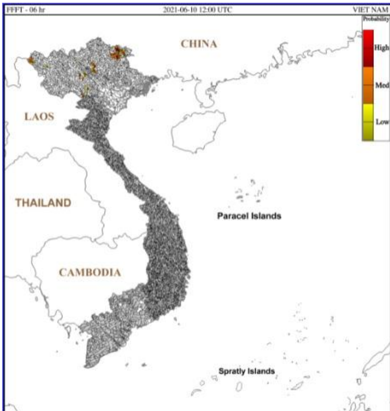
Hình 1. Nguy cơ lũ quét trong 6 giờ tới tại các lưu vực từ 19h ngày 10/06/2021 giờ địa phương
