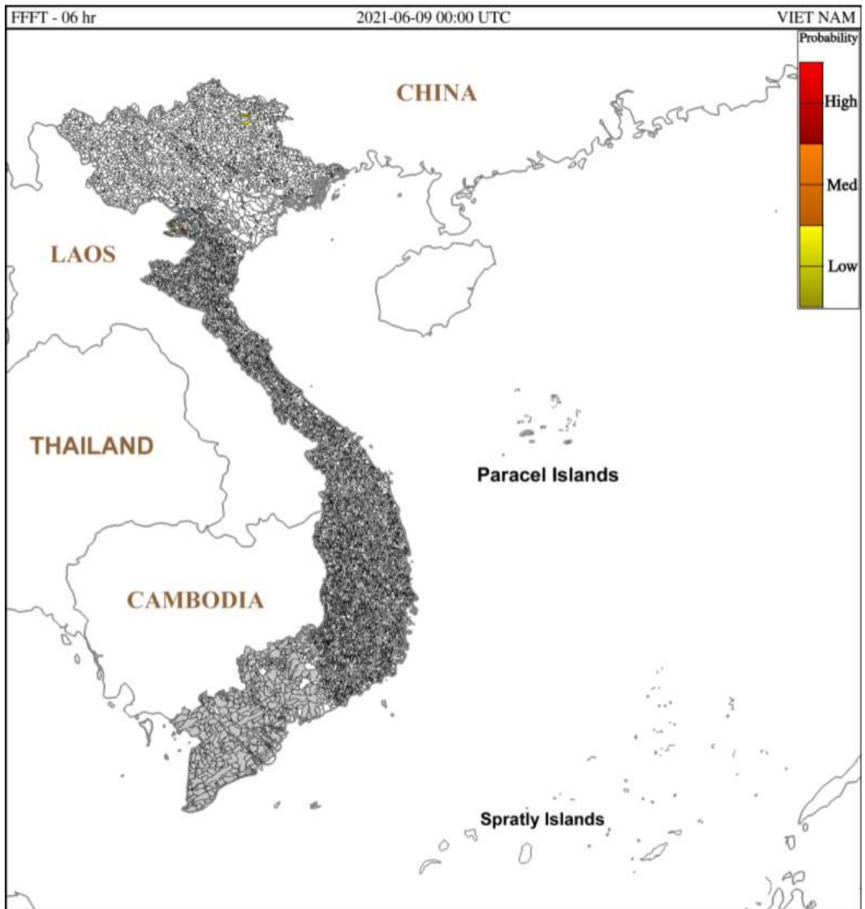
Hình 1. Nguy cơ lũ quét trong 6 giờ tới tại các lưu vực từ 07h ngày 09/06/2021 giờ địa phương
