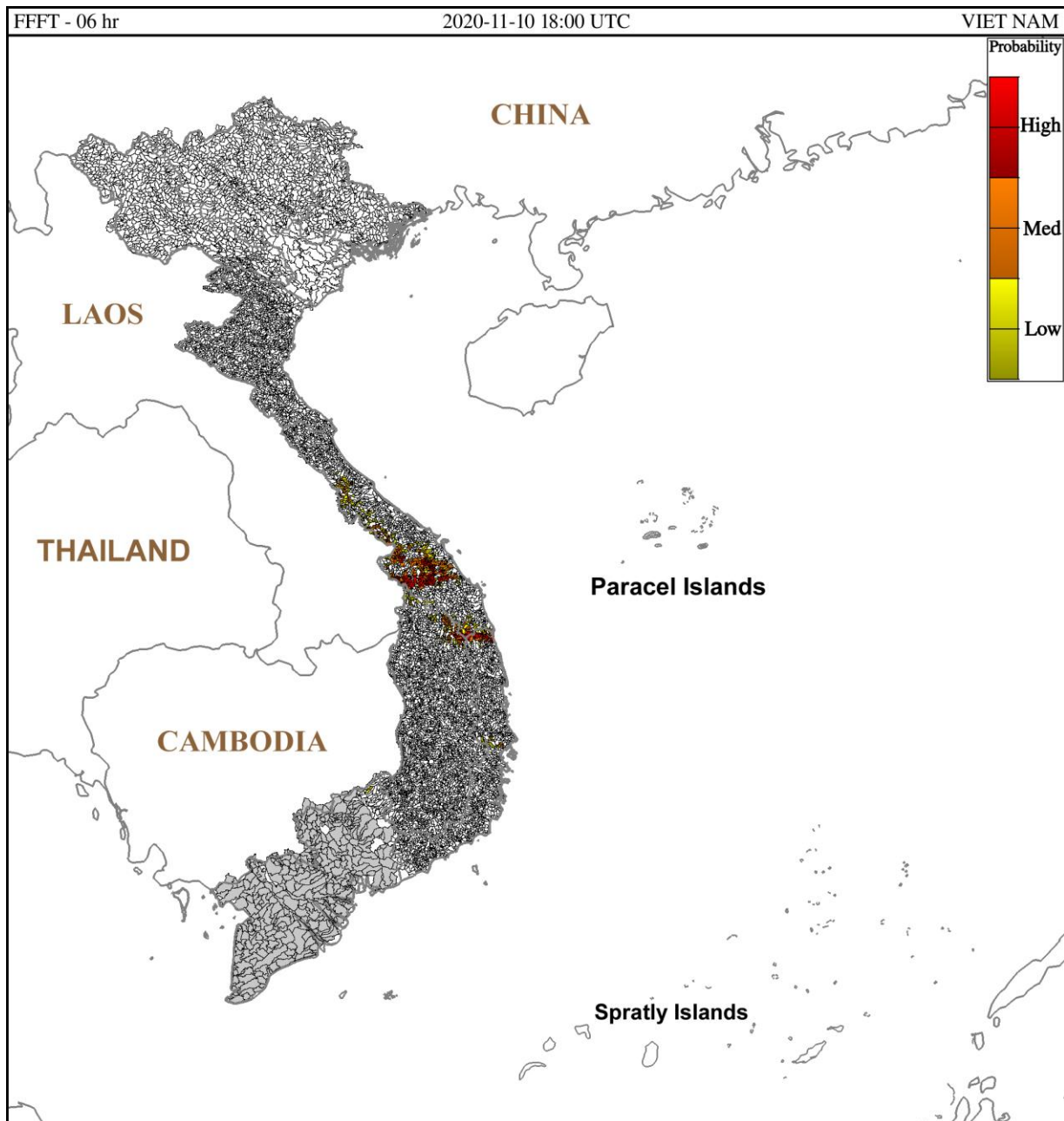
Hình 1. Nguy cơ lũ quét trong 6 giờ tới tại các lưu vực từ 01h ngày 11/11/2020 giờ địa phương
