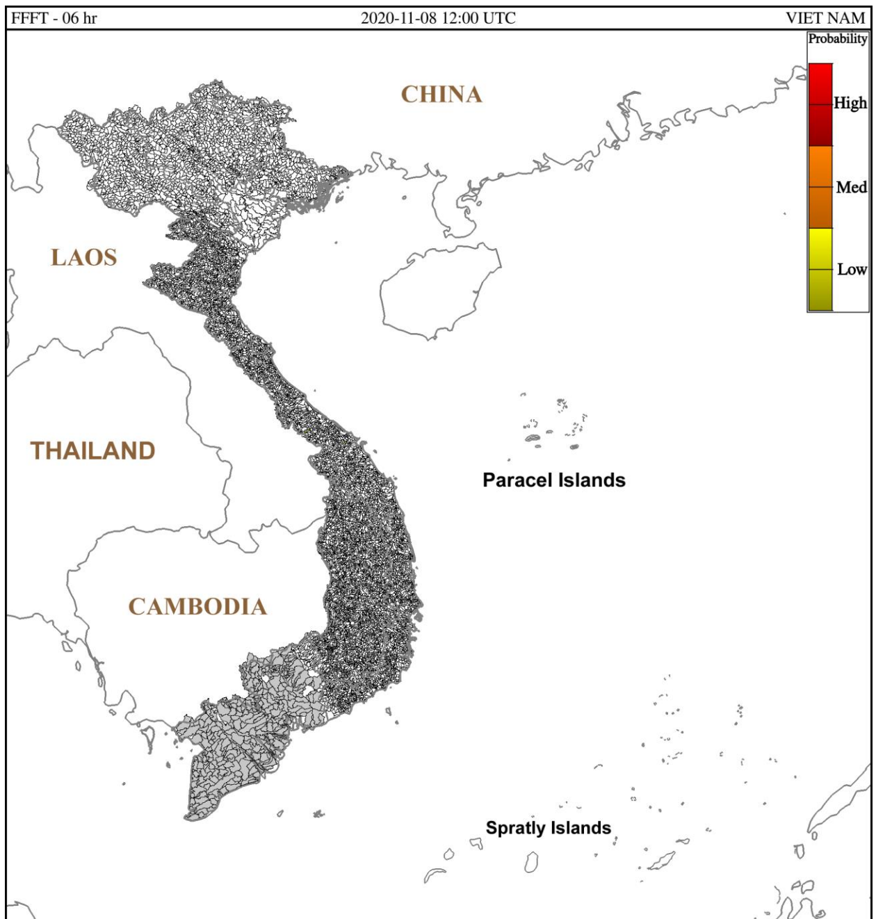
Hình 1. Nguy cơ lũ quét trong 6 giờ tới tại các lưu vực từ 19h ngày 08/11/2020 giờ địa phương
