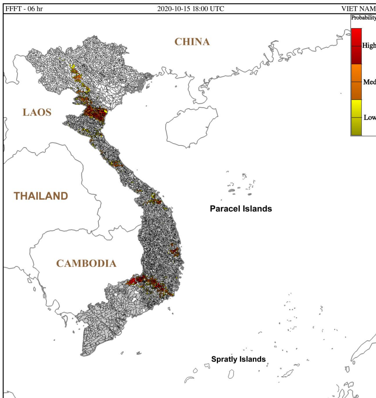
Hình 1. Nguy cơ lũ quét trong 6 giờ tới tại các lưu vực từ 01h ngày 16/10/2020 giờ địa phương
