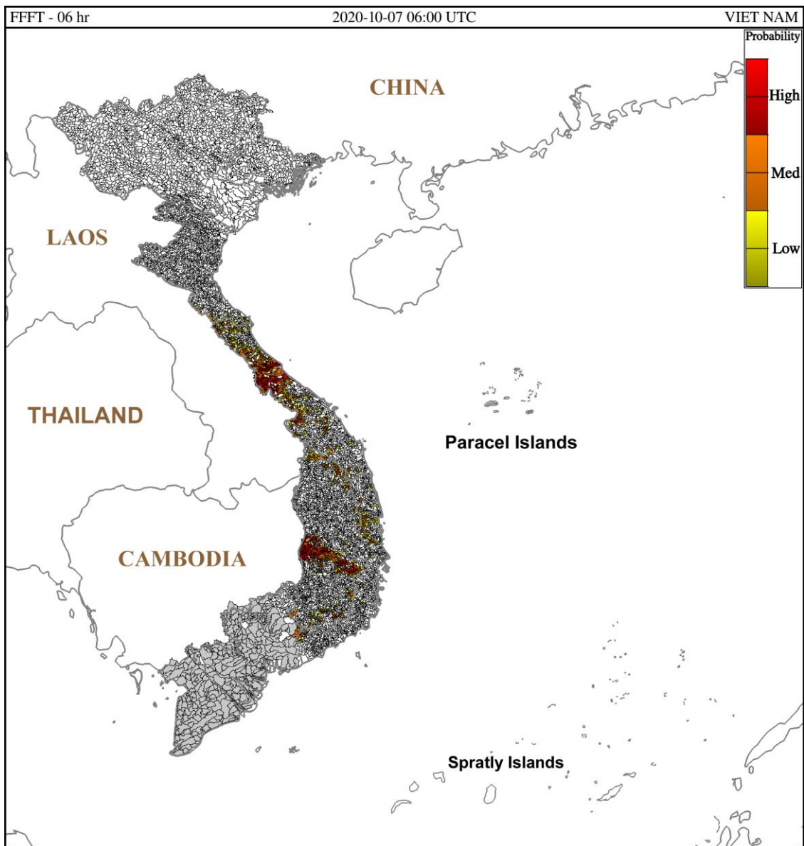
Hình 1: Nguy cơ lũ quét trong 6 giờ tới tại các lưu vực từ 13h ngày 07/10/2020 giờ địa phương
