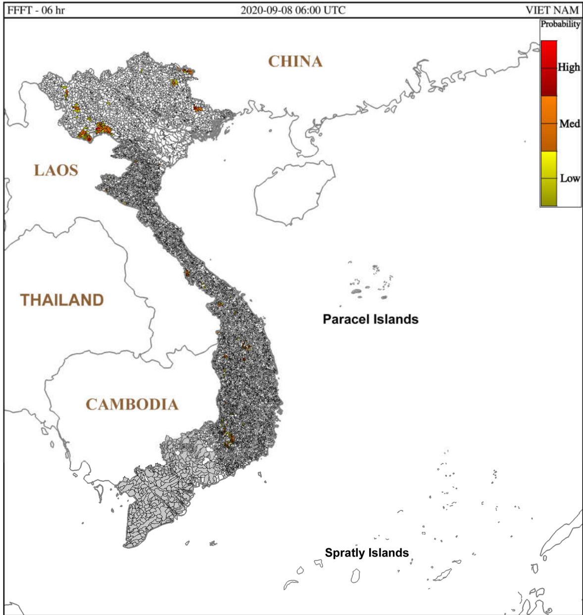
Hình 1. Nguy cơ lũ quét trong 6 giờ tới tại các lưu vực từ 13h ngày 08/9/2020 giờ địa phương
