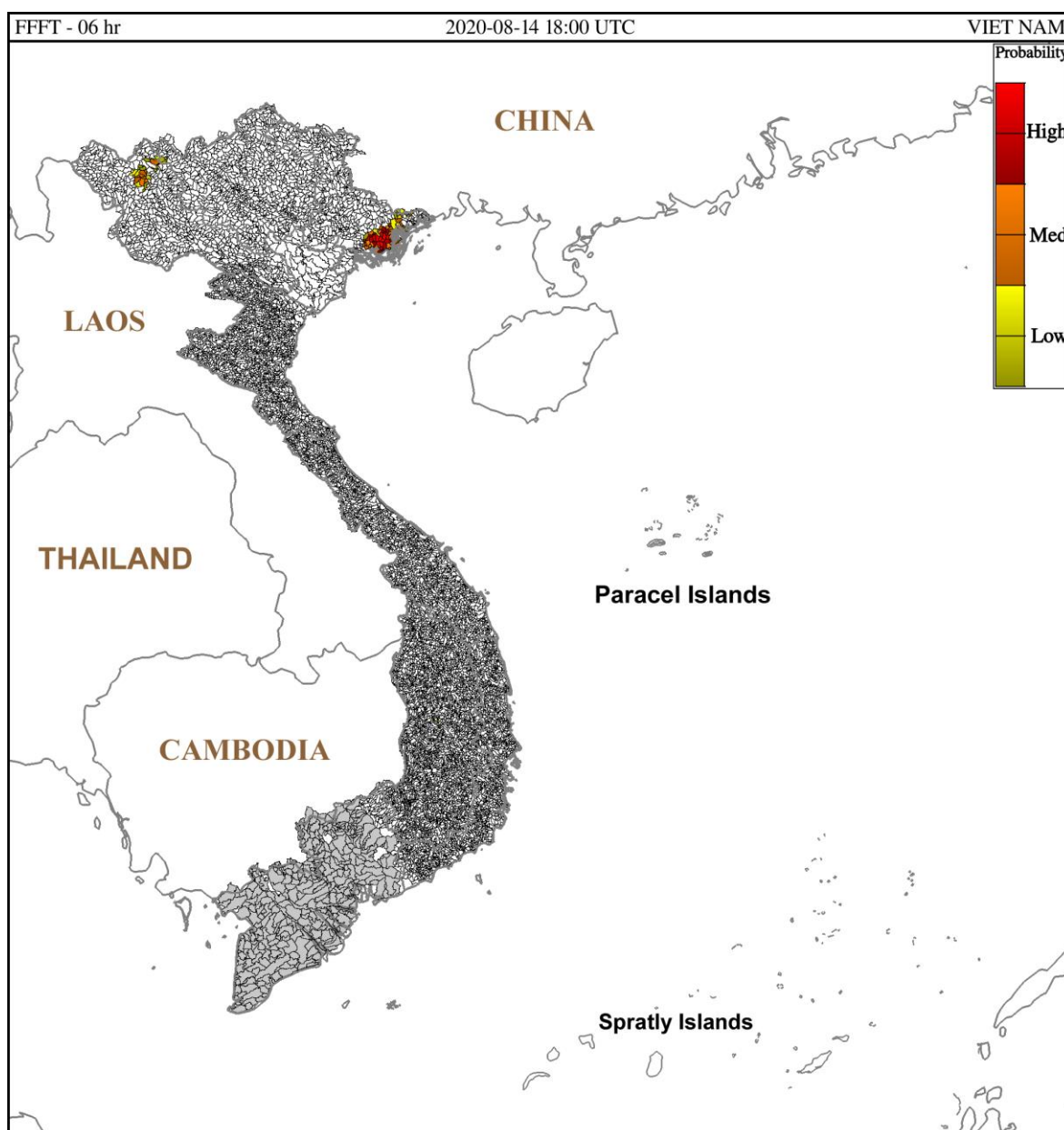
Hình 1: Nguy cơ lũ quét trong 6 giờ tới tại các khu vực từ 01h ngày 15/08/2020 giờ địa phương
