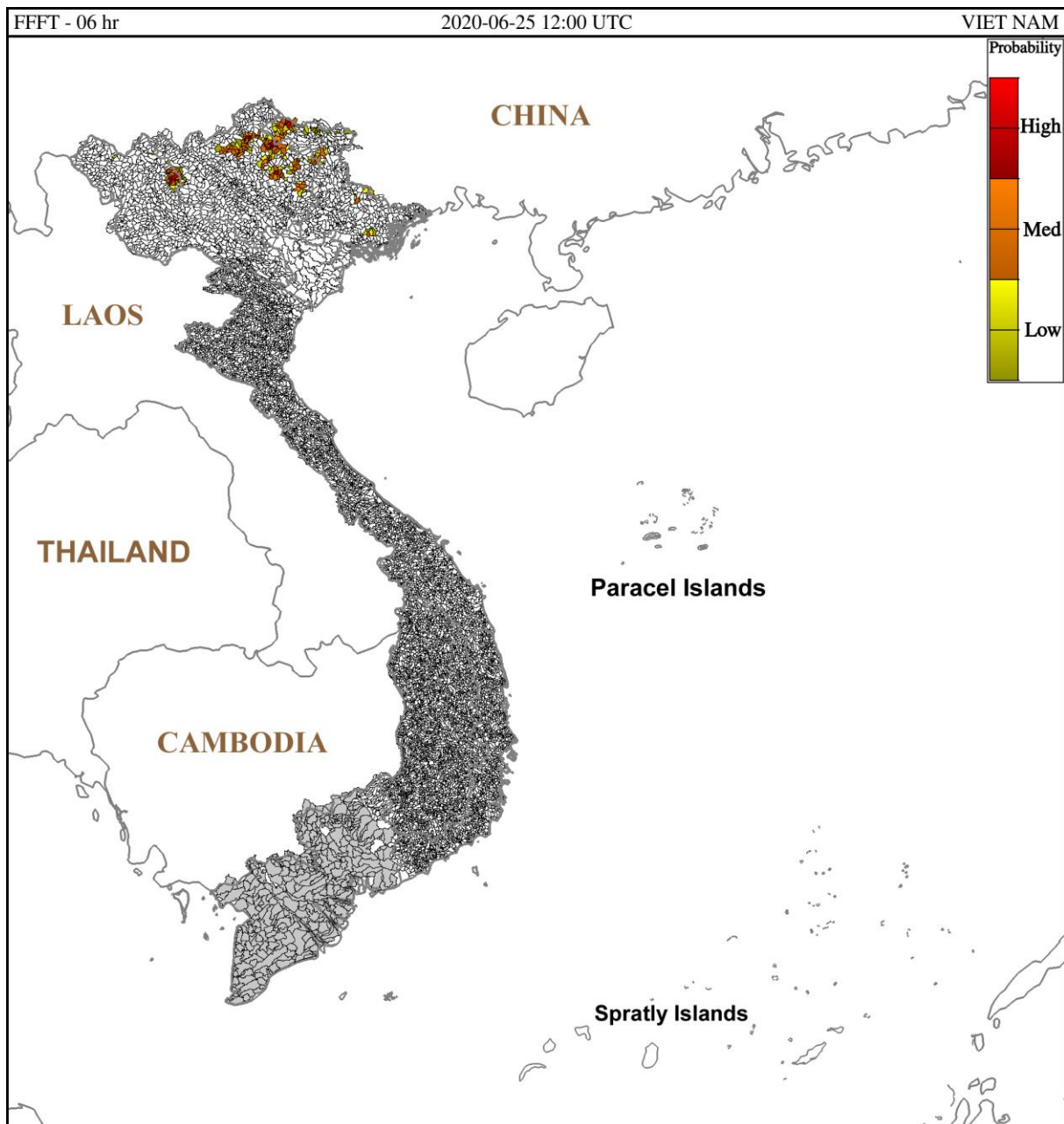
Hình 1: Nguy cơ lũ quét trong 6 giờ tới tại các lưu vực từ 19h ngày 25/06/2020 giờ địa phương
