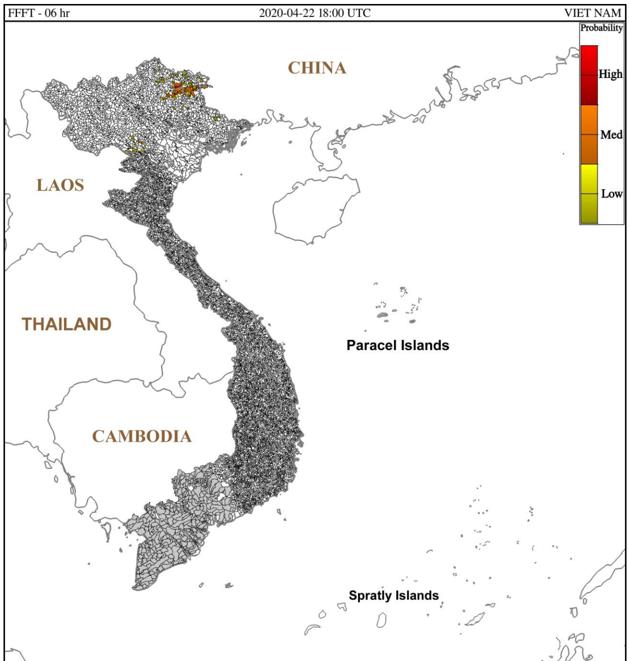
Hình 1: Nguy cơ lũ quét trong 6 giờ tới tại các lưu vực từ 01h ngày 23/04/2020 giờ địa phương
