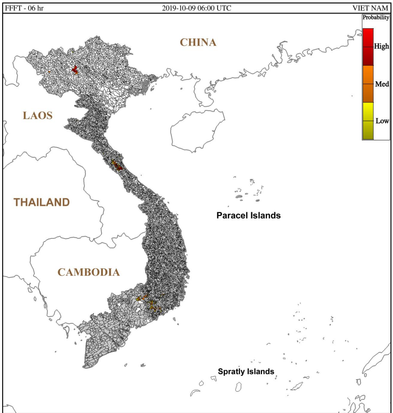
Hình 1. Nguy cơ lũ quét trong 6 giờ tới tại các lưu vực từ 13h ngày 09/10/2019 giờ địa phương
