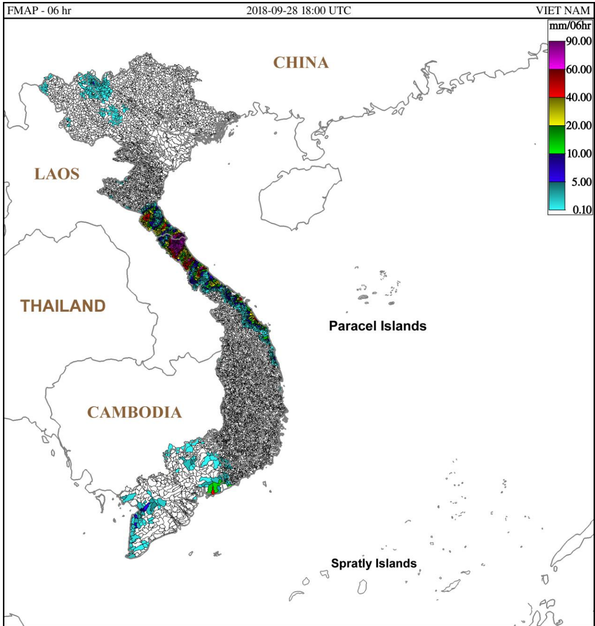
Hình 1: Dự báo lượng mưa trung bình lưu vực 6 giờ tính từ 01h ngày 29/09/2018 giờ địa phương
