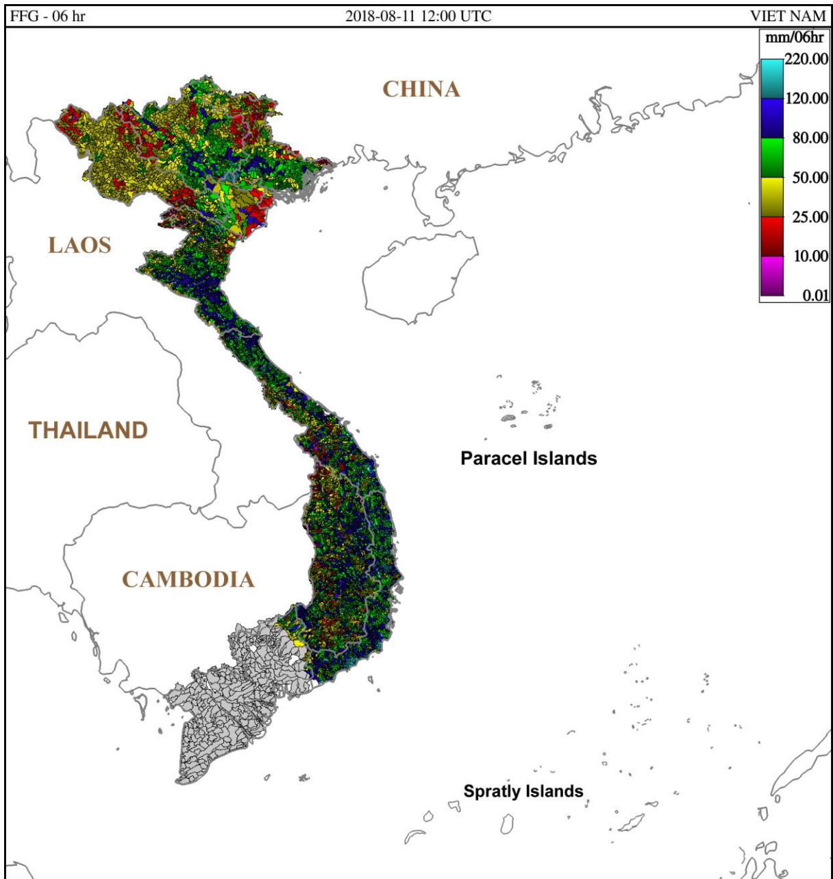
Hình 1. Ngưỡng mưa định hướng có khả năng sinh lũ quét trong 6 giờ tới tại các lưu vực từ 19h ngày 11/08/2018 giờ địa phương
