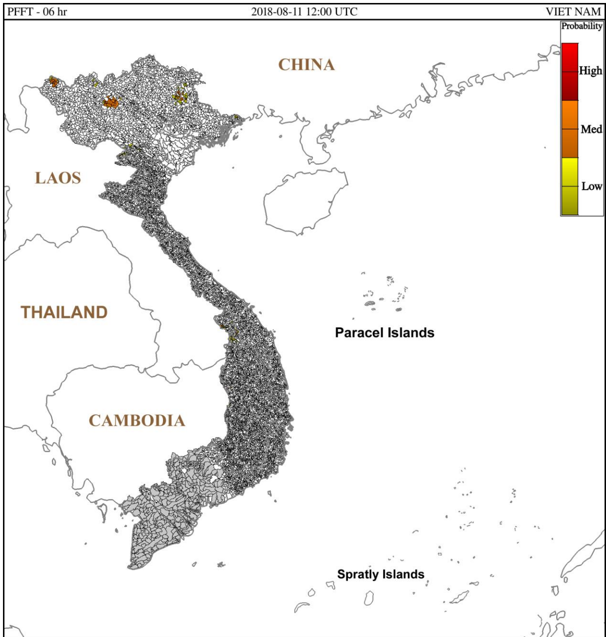
Hình 3: Nguy cơ lũ quét trong 6 giờ tới tại các lưu vực từ 19h ngày 11/08/2018 giờ địa phương
