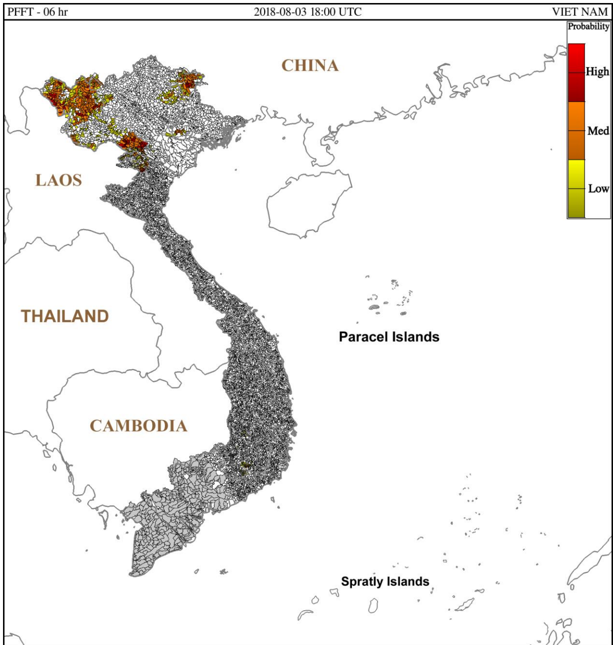
Hình 3: Nguy cơ lũ quét trong 6 giờ tới tại các lưu vực từ 01h ngày 04/08/2018 giờ địa phương
