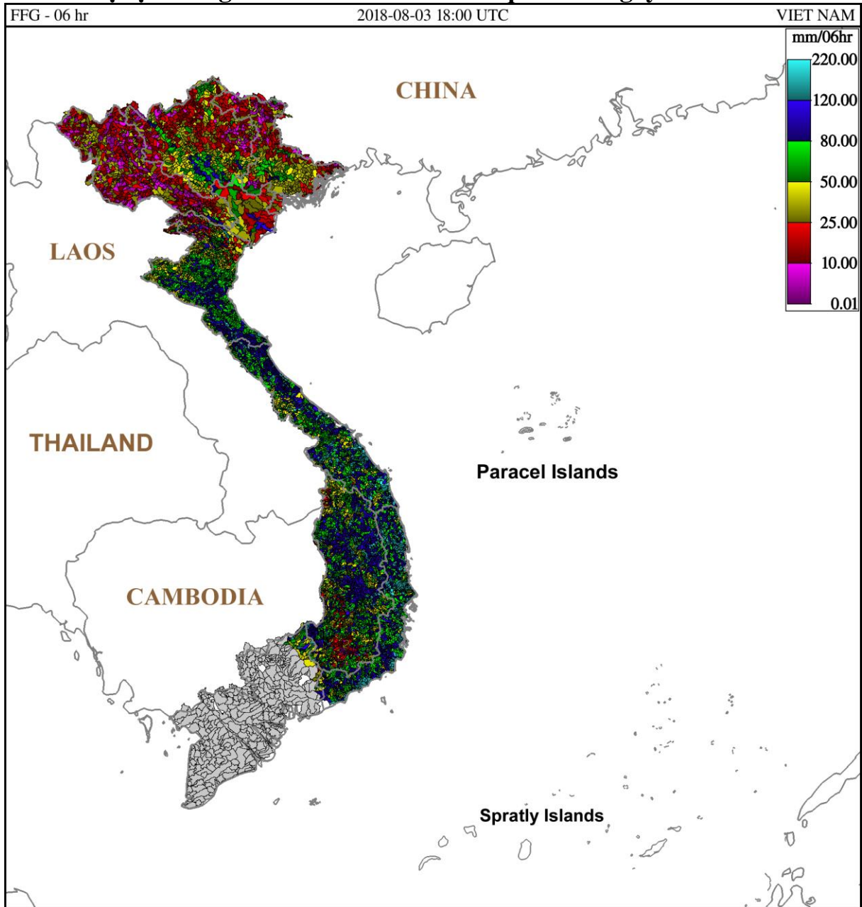
Hình 1. Ngưỡng mưa định hướng có khả năng sinh lũ quét trong 6 giờ tới tại các lưu vực từ 01h ngày 04/08/2018 giờ địa phương
