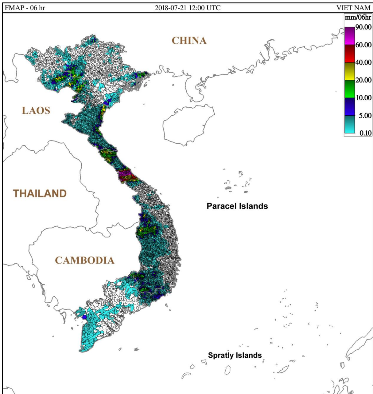
Hình 2: Dự báo lượng mưa trung bình lưu vực 6 giờ tính từ 19h ngày 21/07/2018 giờ địa phương
