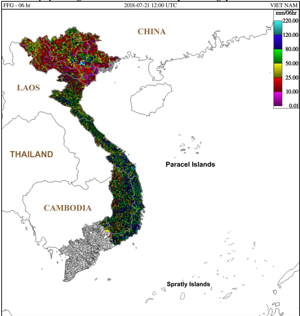
Hình 1: Ngưỡng mưa định hướng có khả năng sinh lũ quét trong 6 giờ tới tại các lưu vực từ 19h ngày 21/07/2018 giờ địa phương
