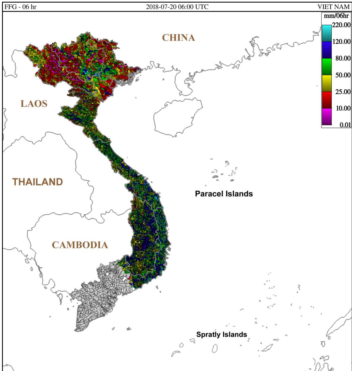
Hình 1. Ngưỡng mưa định hướng có khả năng sinh lũ quét trong 6 giờ tới tại các lưu vực từ 13h ngày 20/07/2018 giờ địa phương
