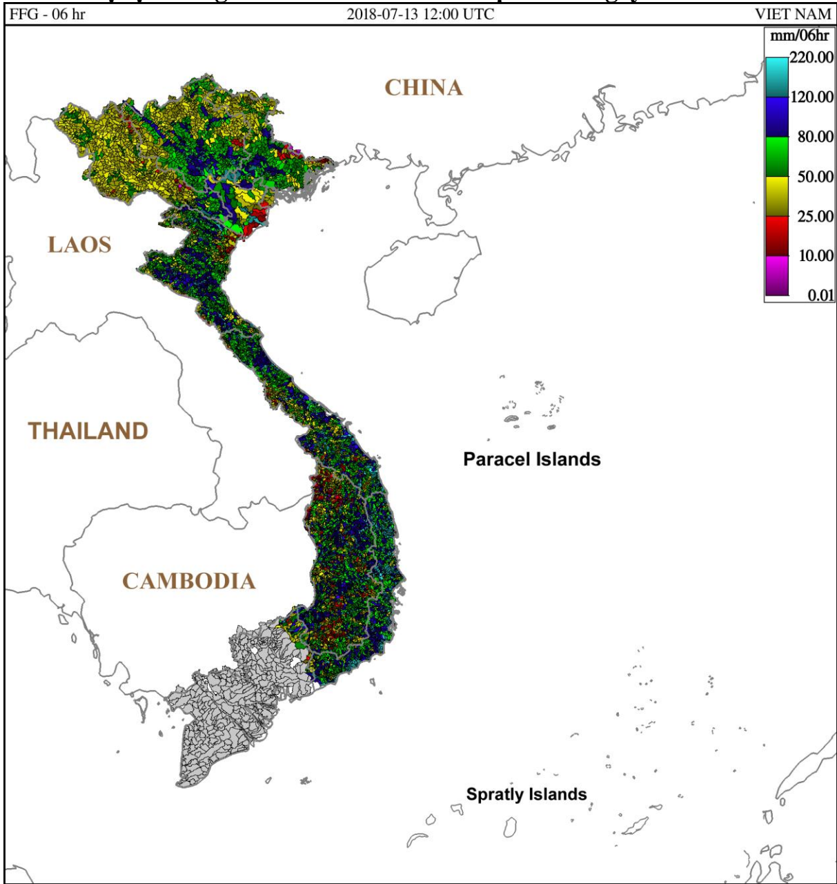
Hình 1. Ngưỡng mưa định hướng có khả năng sinh lũ quét trong 6 giờ tới tại các lưu vực từ 19h ngày 13/07/2018 giờ địa phương
