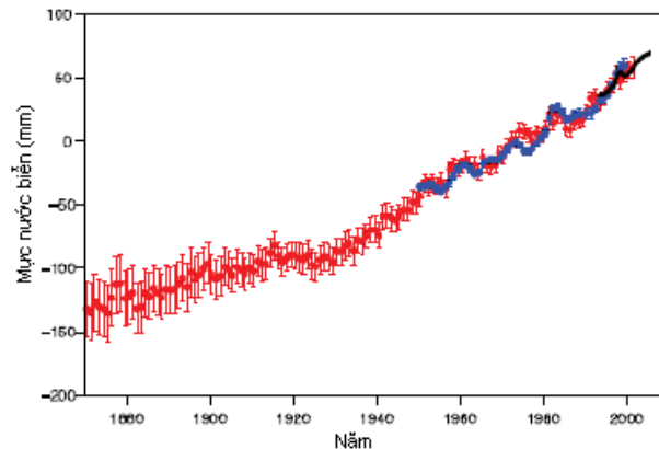
Hình 3. Diễn biến của mực nước biển trung bình toàn cầu. Nguồn: IPCC/2007
