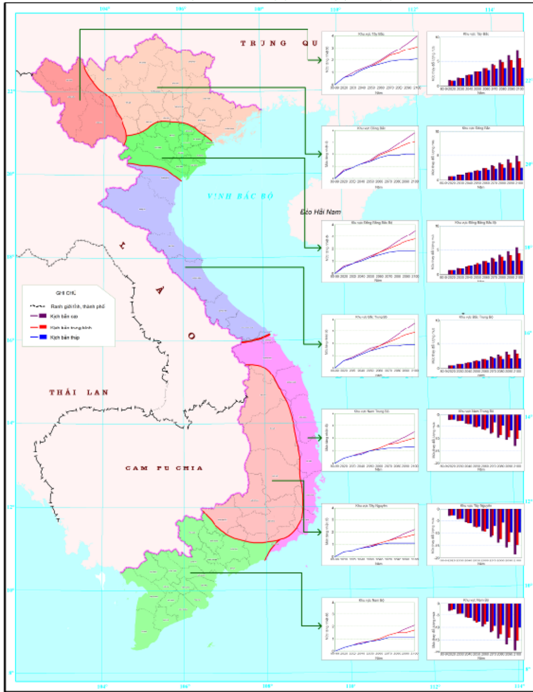
Phụ lục 1. Mức tăng nhiệt độ trung bình (°C) và mức thay đổi lượng mưa (%) vào các tháng XII-II so với trung bình thời kỳ 1980-1999 ở các vùng khí hậu của Việt ả am theo các kịch bản phát thải thấp (B1), trung bình (B2) và cao (A2)
