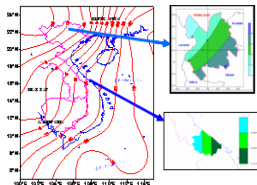
Hình 12. Kịch bản biến đổi khí hậu cho Việt ả am và các khu vực nhỏ hơn
