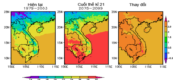
Hình 10. Sản phẩm mô phỏng nhiệt độ của mô hình MRI-AGCM cho khu vực Việt ấu am
