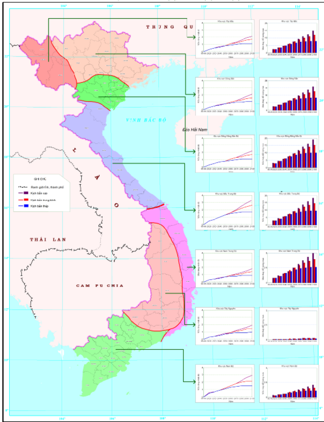
Phụ lục 3. Mức tăng nhiệt độ trung bình (°C) và mức thay đổi lượng mưa (%) vào các tháng VI-VIII so với trung bình thời kỳ 1980-1999 ở các vùng khí hậu của Việt ả am theo các kịch bản phát thải thấp (B1), trung bình (B2) và cao (A2)
