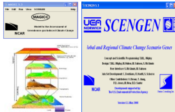
Hình 14. Phần mềm MAGICC/SCEA GE 5.3 và phương pháp chi tiết hóa thống kê
