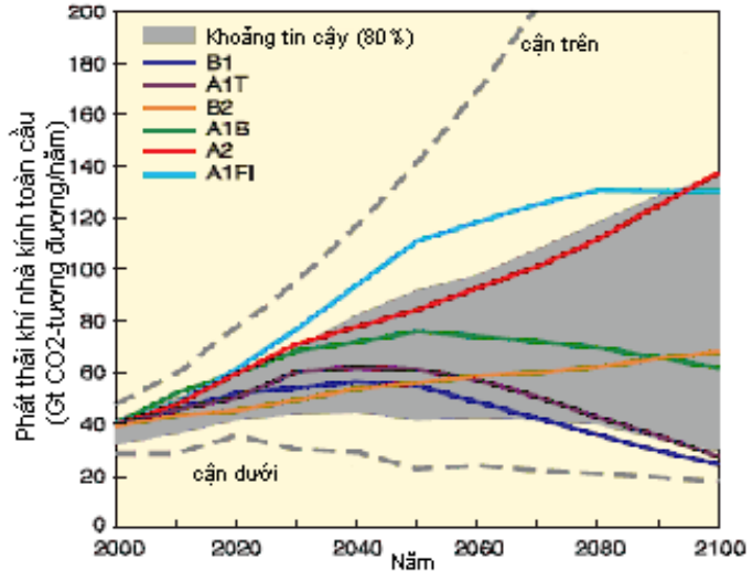
Hình 8. Lượng phát thải CO 2 tương đương trong thế kỷ 21 của các kịch bản. ấu nguồn: IPCC
