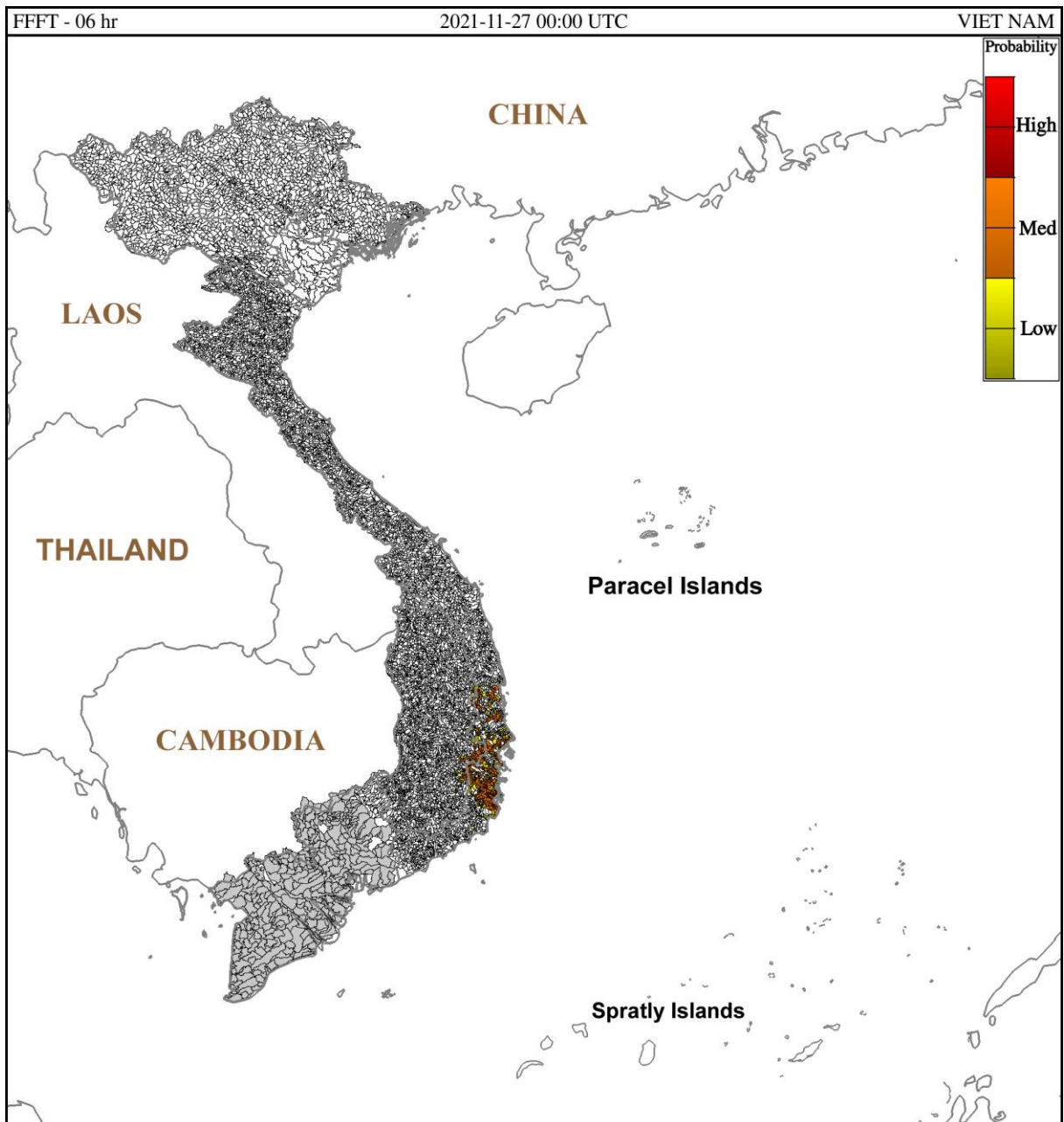
Hình 1. Nguy cơ lũ quét trong 6 giờ tới tại các lưu vực từ 07h ngày 27/11/2021 giờ địa phương
