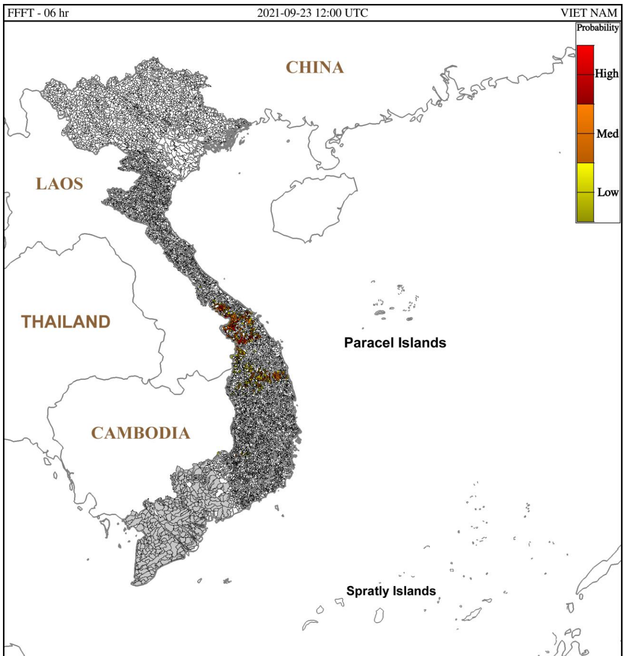
Hình 1. Nguy cơ lũ quét trong 6 giờ tới tại các lưu vực từ 19h ngày 23/9/2021 giờ địa phương
