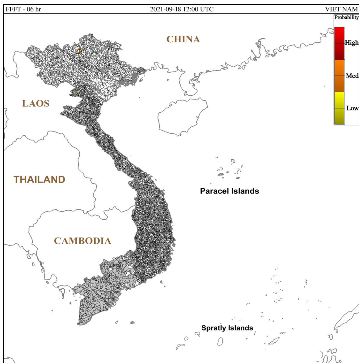
Hình 1. Nguy cơ lũ quét trong 6 giờ tới tại các lưu vực từ 19h ngày 18/09/2021 giờ địa phương
