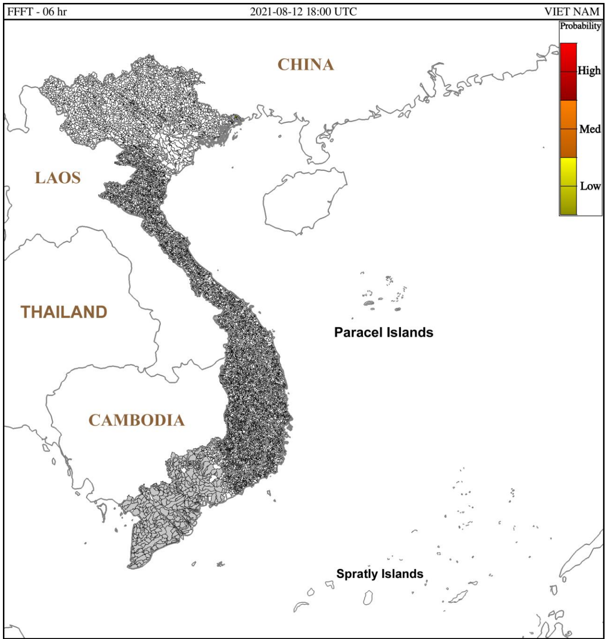
Hình 1. Nguy cơ lũ quét trong 6 giờ tới tại các lưu vực từ 01h ngày 13/08/2021 giờ địa phương
