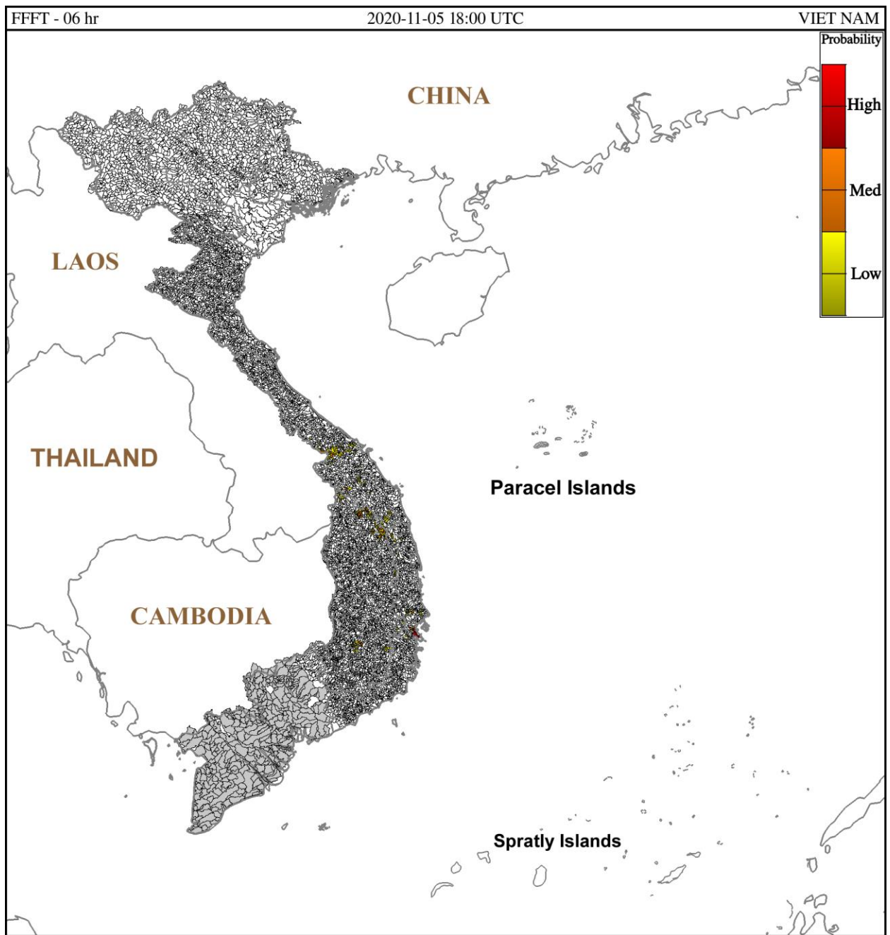
Hình 1. Nguy cơ lũ quét trong 6 giờ tới tại các lưu vực từ 01h ngày 06/11/2020 giờ địa phương
