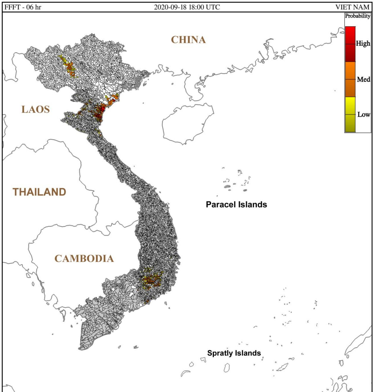
Hình 1. Nguy cơ lũ quét trong 6 giờ tới tại các lưu vực từ 01h ngày 19/9/2020 giờ địa phương
