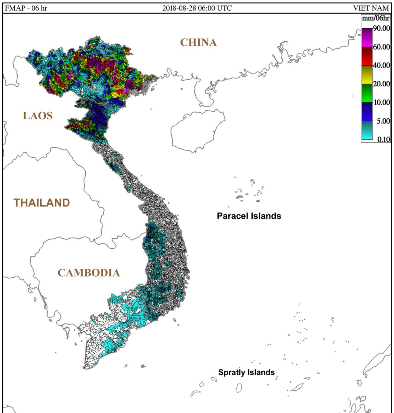
Hình 1: Dự báo lượng mưa trung bình lưu vực 6 giờ tính từ 13h ngày 28-08-2018 giờ địa phương
