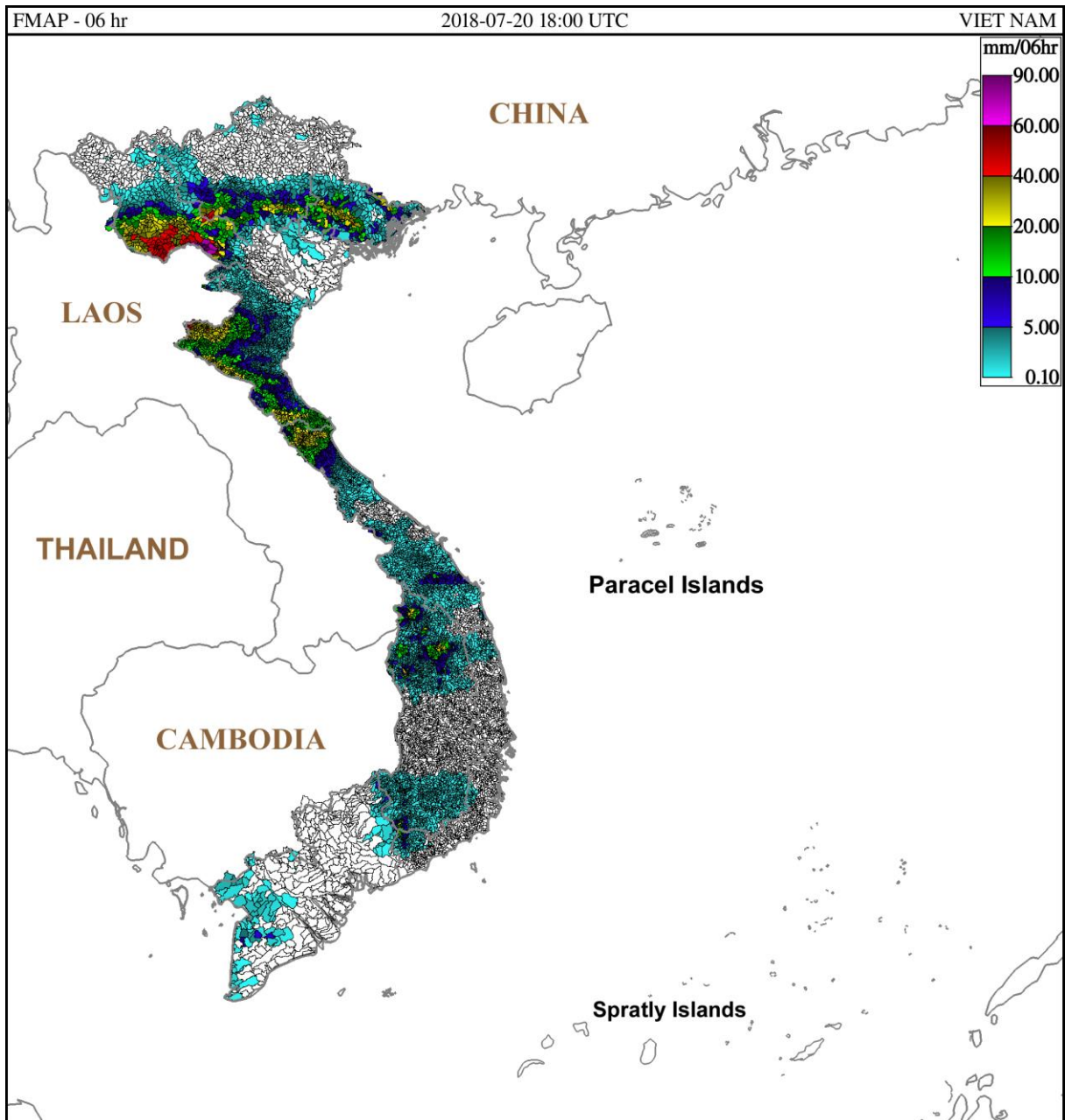
Hình 2: Dự báo lượng mưa trung bình lưu vực 6 giờ tính từ 01h ngày 21/07/2018 giờ địa phương
