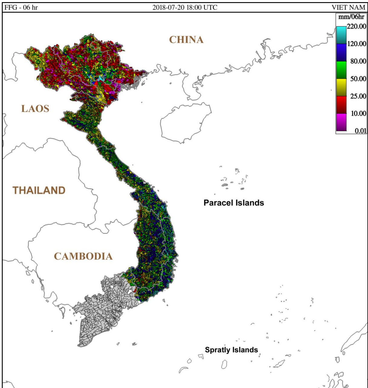
Hình 1. Ngưỡng mưa định hướng có khả năng sinh lũ quét trong 6 giờ tới tại các lưu vực từ 01h ngày 21/07/2018 giờ địa phương
