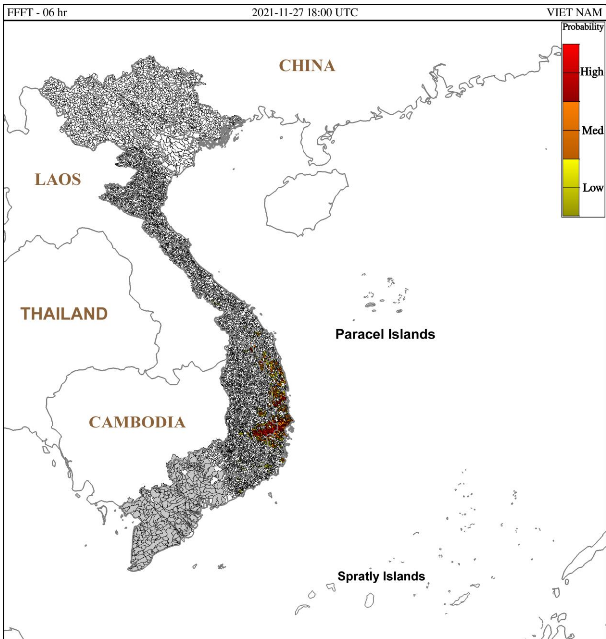
Hình 1. Nguy cơ lũ quét trong 6 giờ tới tại các lưu vực từ 01h ngày 28/11/2021 giờ địa phương
