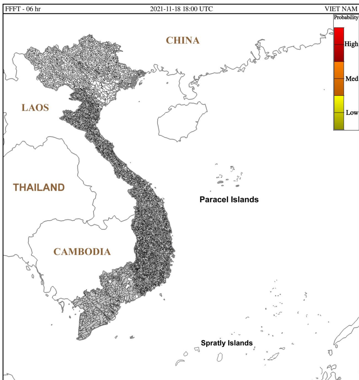
Hình 1. Nguy cơ lũ quét trong 6 giờ tới tại các lưu vực từ 01h ngày 19/11/2021 giờ địa phương
