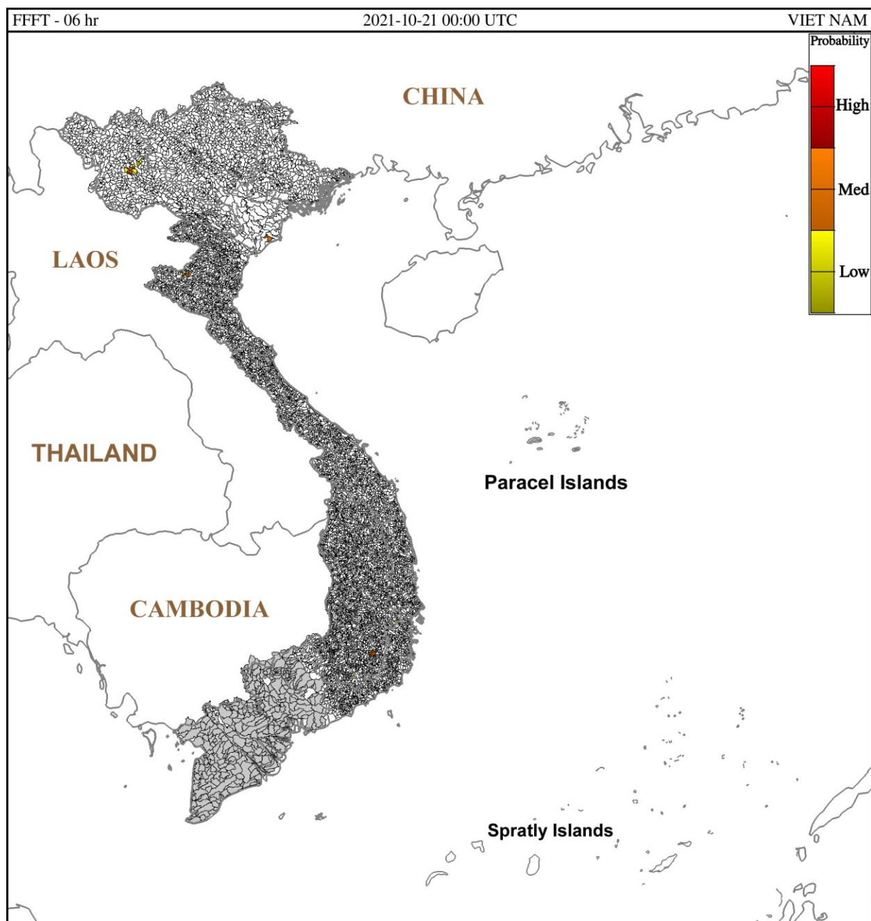
Hình 1. Nguy cơ lũ quét trong 6 giờ tới tại các lưu vực từ 07h ngày 21/10/2021 giờ địa phương
