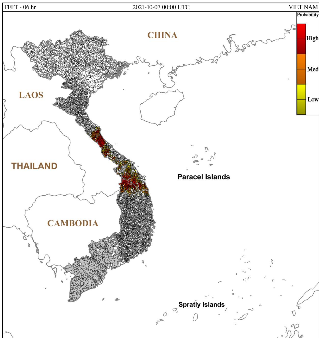
Hình 1. Nguy cơ lũ quét trong 6 giờ tới tại các lưu vực từ 07h ngày 07/10/2021 giờ địa phương
