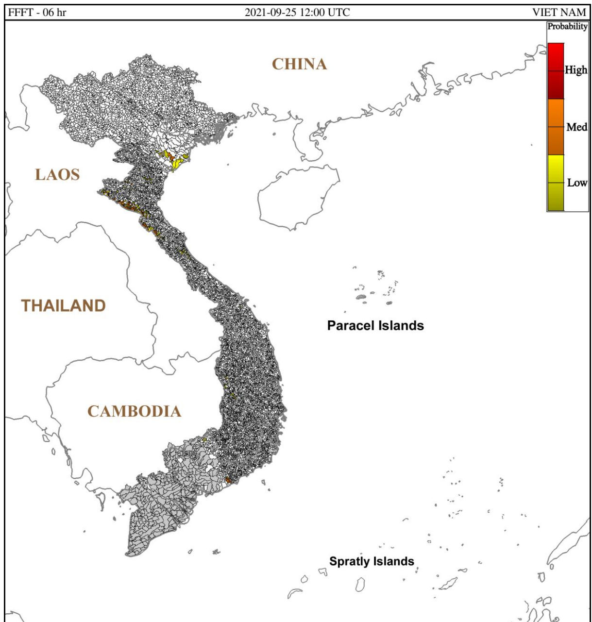
Hình 1. Nguy cơ lũ quét trong 6 giờ tới tại các lưu vực từ 19h ngày 25/09/2021 giờ địa phương
