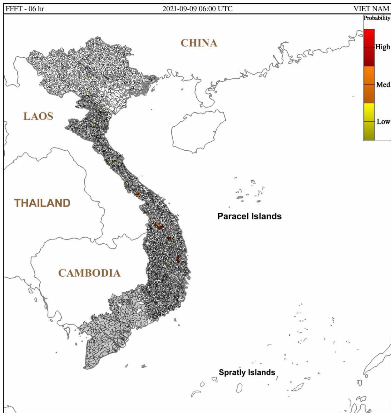
Hình 1. Nguy cơ lũ quét trong 6 giờ tới tại các lưu vực từ 13h ngày 09/9/2021 giờ địa phương
