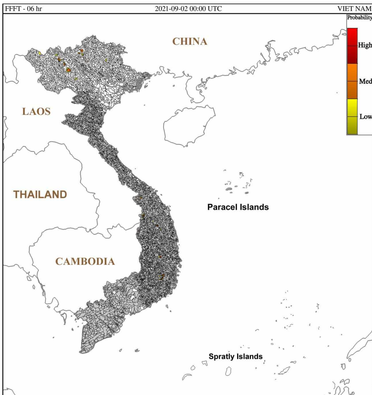
Hình 1. Nguy cơ lũ quét trong 6 giờ tới tại các lưu vực từ 07h ngày 02/9/2021 giờ địa phương
