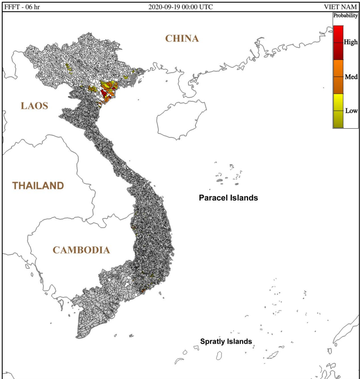
Hình 1. Nguy cơ lũ quét trong 6 giờ tới tại các lưu vực từ 07h ngày 19/09/2020 giờ địa phương
