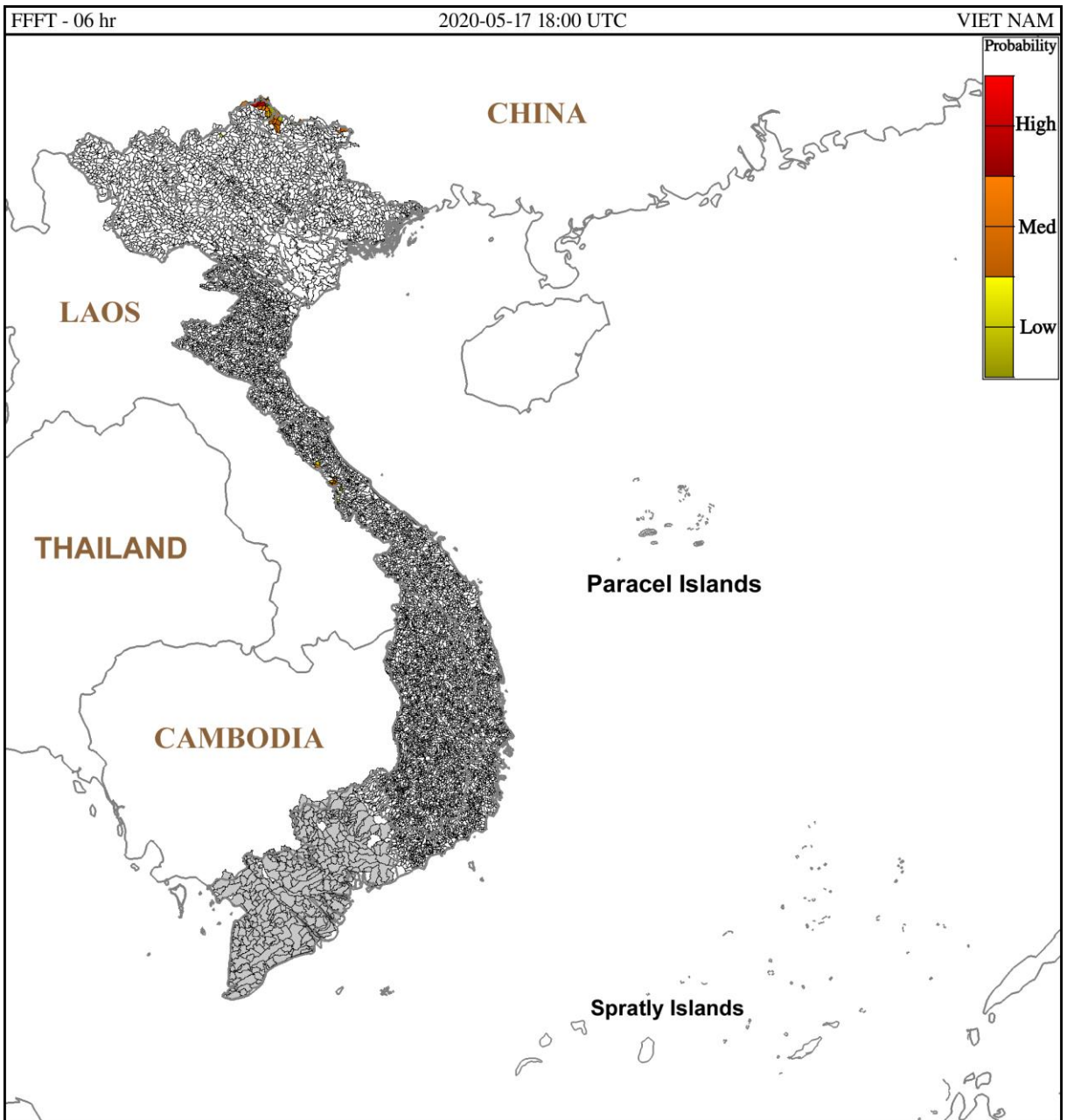
Hình 1. Nguy cơ lũ quét trong 6 giờ tới tại các lưu vực từ 01h ngày 18/05/2020 giờ địa phương
