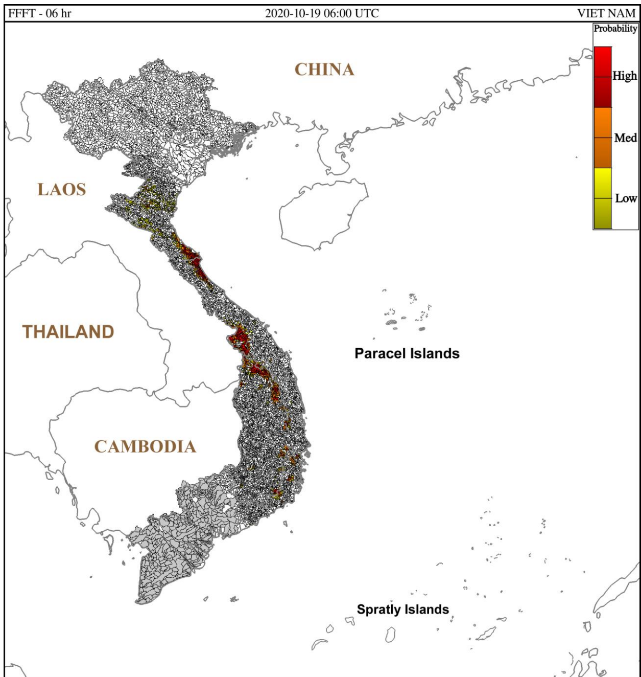
Hình 1. Nguy cơ lũ quét trong 6 giờ tới tại các lưu vực từ 13h ngày 19/10/2020 giờ địa phương
