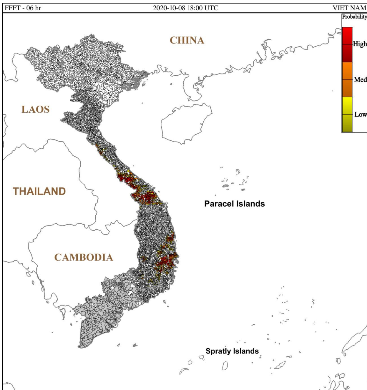
Hình 1. Nguy cơ lũ quét trong 6 giờ tới tại các lưu vực từ 01h ngày 09/10/2020 giờ địa phương
