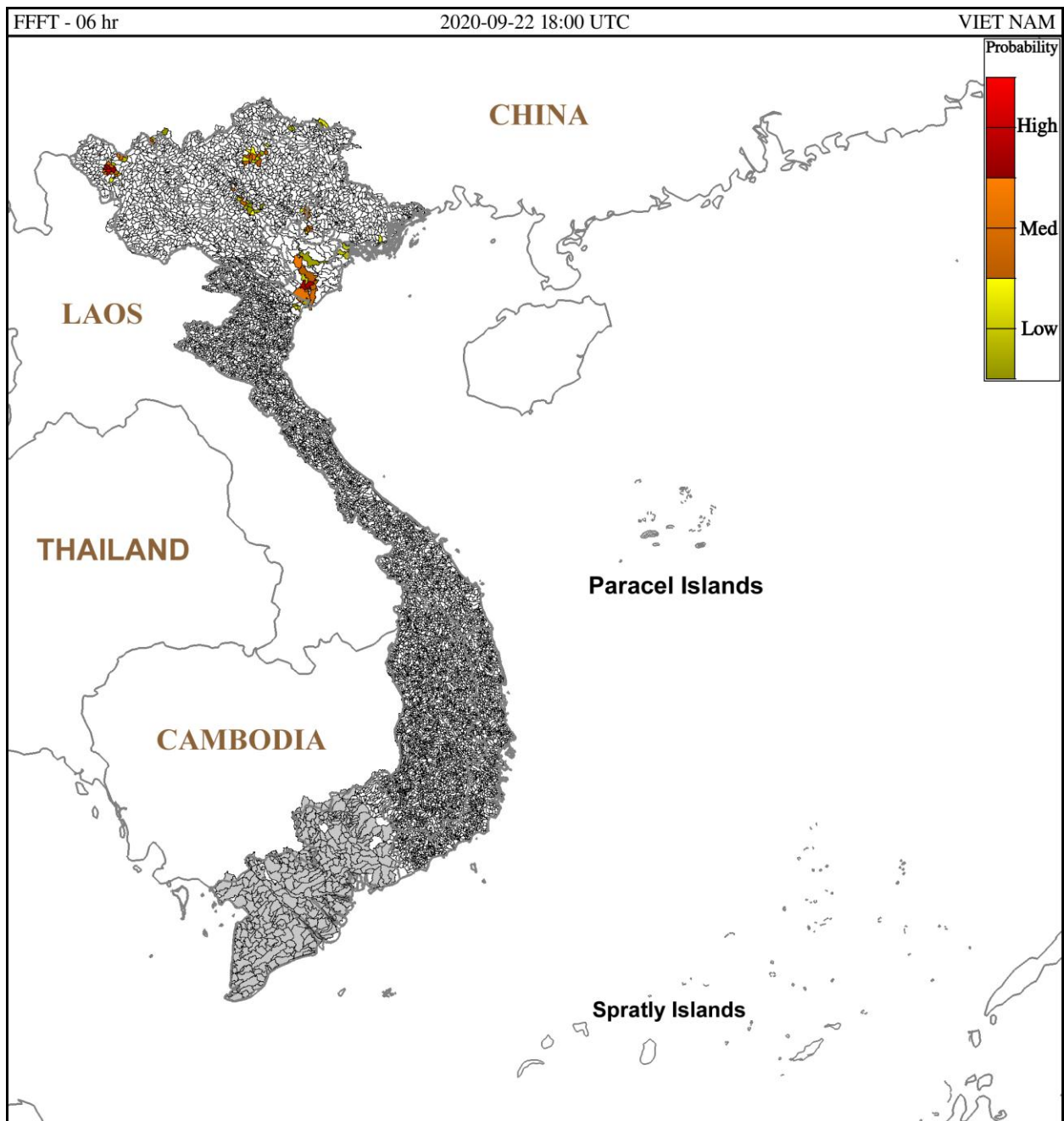
Hình 1. Nguy cơ lũ quét trong 6 giờ tới tại các lưu vực từ 01h ngày 23/9/2020 giờ địa phương
