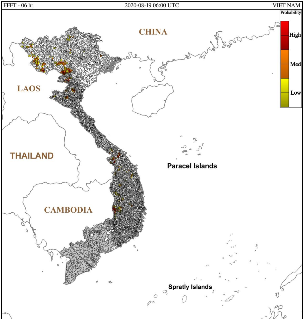
Hình 1. Nguy cơ lũ quét trong 6 giờ tới tại các lưu vực từ 13h ngày 19/08/2020 giờ địa phương
