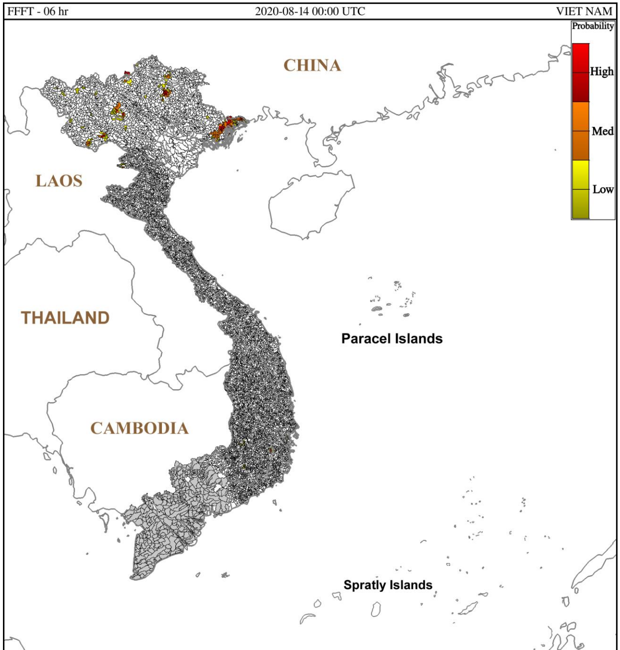
Hình 1: Nguy cơ lũ quét trong 6 giờ tới tại các khu vực từ 07h ngày 14/08/2020 giờ địa phương
