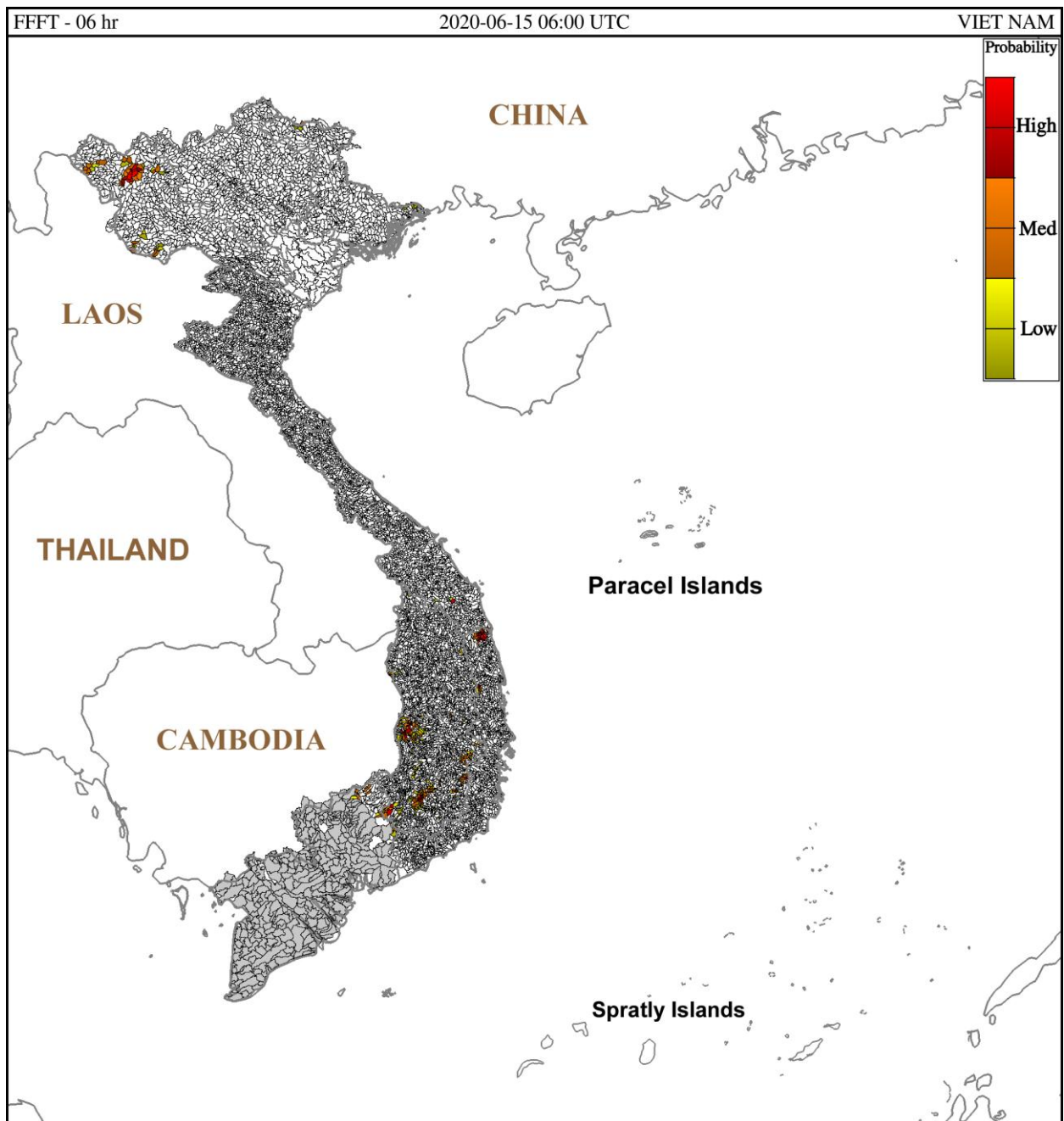
Hình 1: Nguy cơ lũ quét trong 6 giờ tới tại các khu vực từ 13h ngày 15/6/2020 giờ địa phương
