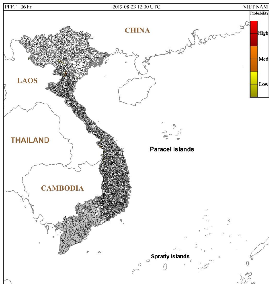
Hình 1: Nguy cơ lũ quét trong 6 giờ tới tại các lưu vực từ 19h ngày 23/08/2019 giờ địa phương
