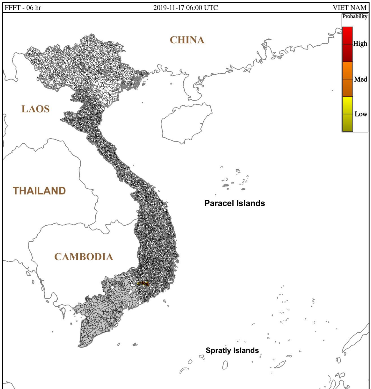
Hình 1. Nguy cơ lũ quét trong 6 giờ tới tại các lưu vực từ 13h ngày 17/11/2019 giờ địa phương
