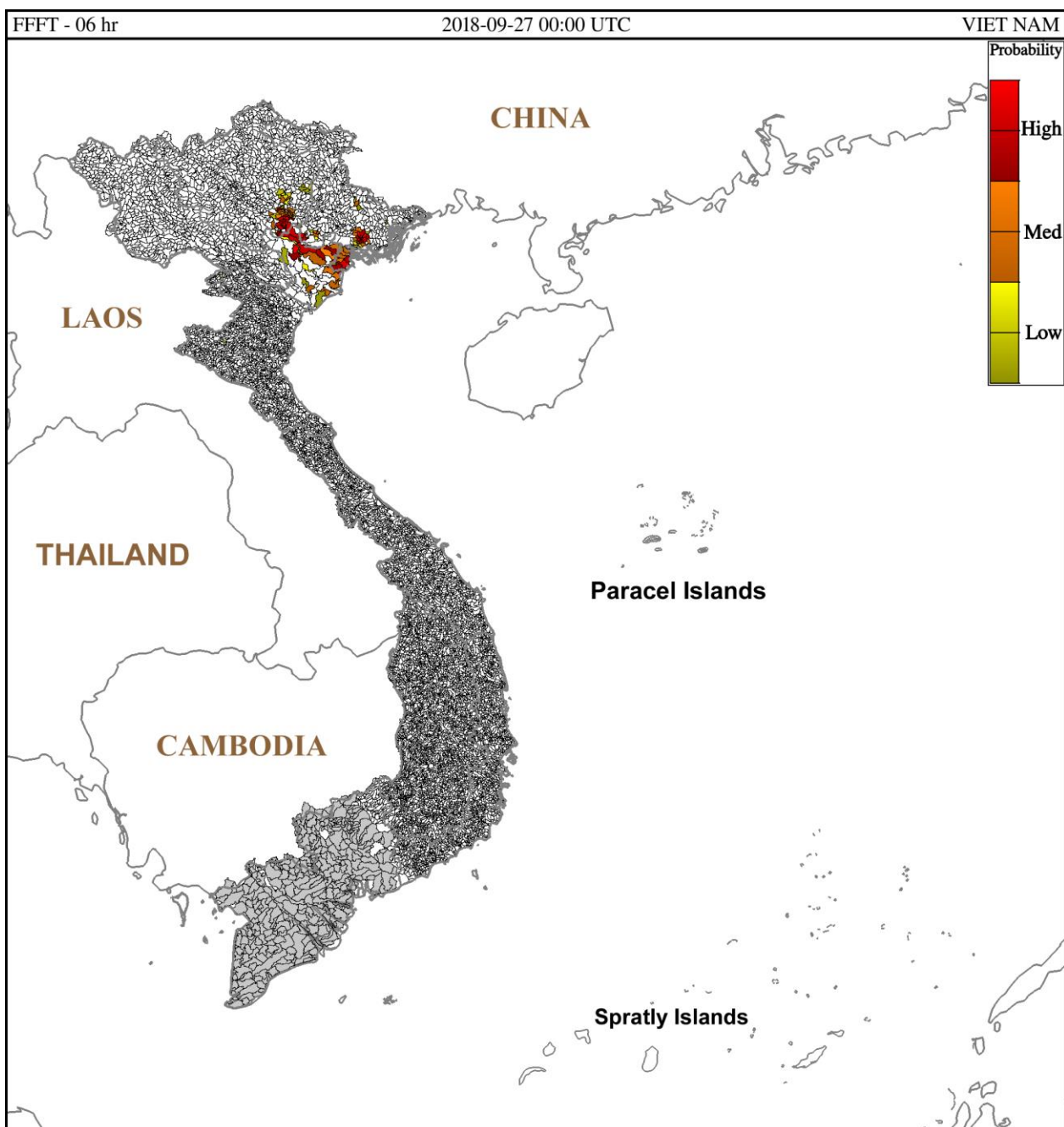
Hình 2: Nguy cơ lũ quét trong 6 giờ tới tại các lưu vực từ 07h ngày 27-09-2018 giờ địa phương
