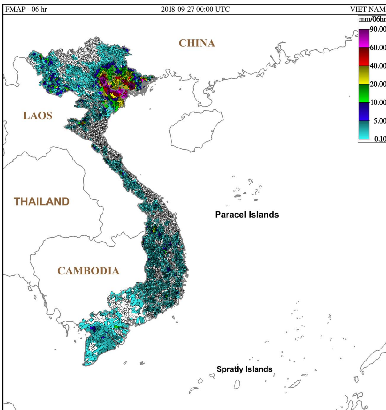
Hình 1: Dự báo lượng mưa trung bình lưu vực 6 giờ tính từ 07h ngày 27-09-2018 giờ địa phương
