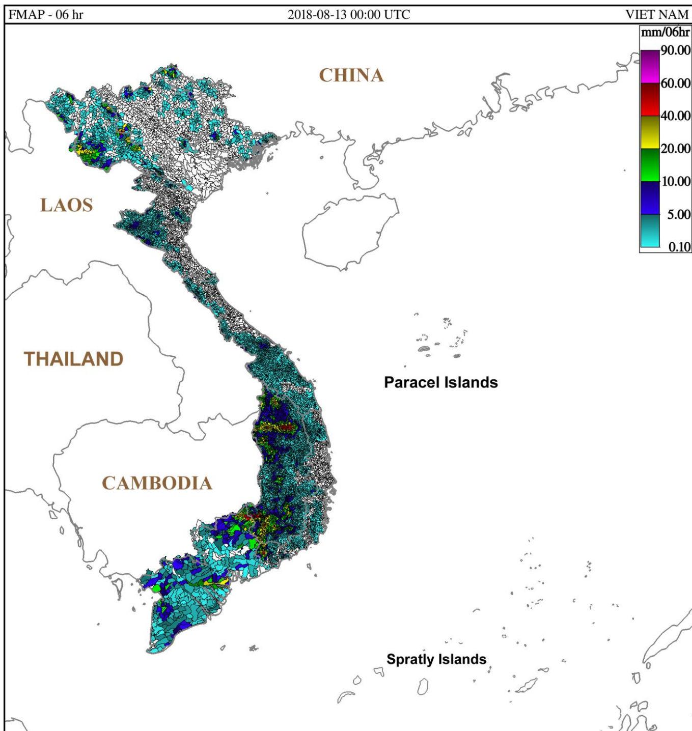
Hình 2: Dự báo lượng mưa trung bình lưu vực 6 giờ tính từ 07h ngày 13/08/2018 giờ địa phương
