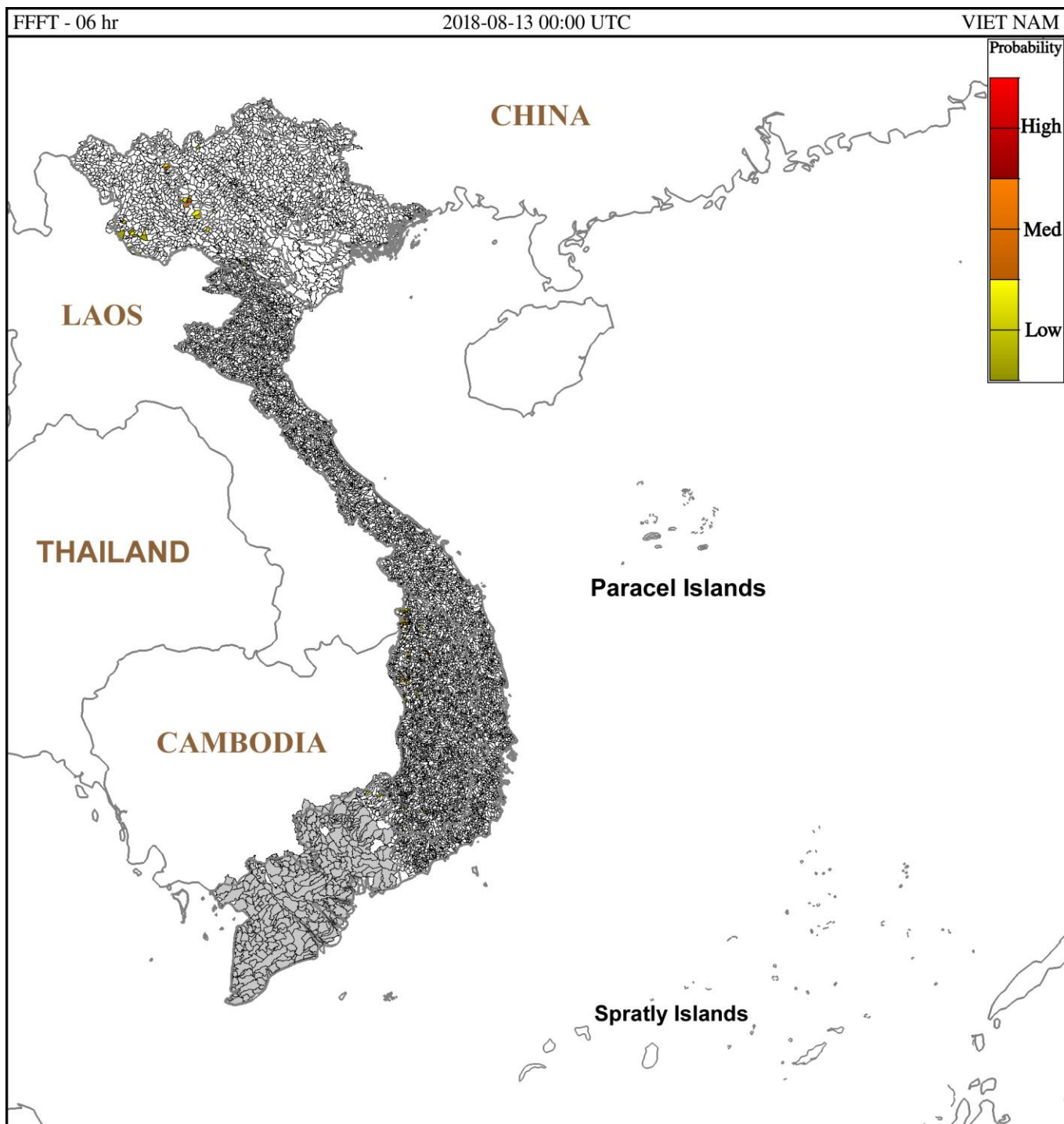
Hình 3: Nguy cơ lũ quét trong 6 giờ tới tại các lưu vực từ 07h ngày 13/08/2018 giờ địa phương
