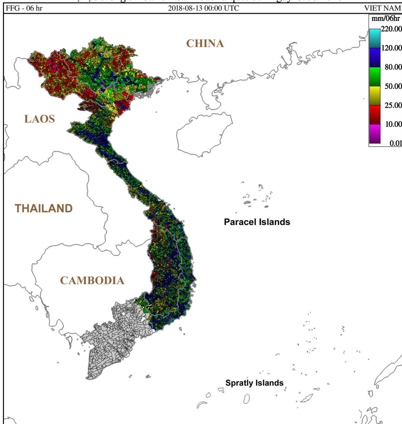
Hình 1. Ngưỡng mưa định hướng có khả năng sinh lũ quét trong 6 giờ tới tại các lưu vực từ 07h ngày 13/08/2018 giờ địa phương
