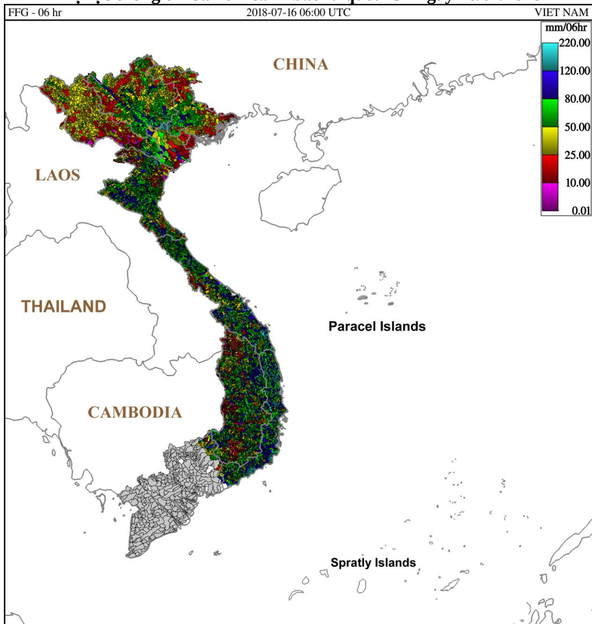
Hình 1. Ngưỡng mưa định hướng có khả năng sinh lũ quét trong 6 giờ tới tại các lưu vực từ 13h ngày 16/07/2018 giờ địa phương
