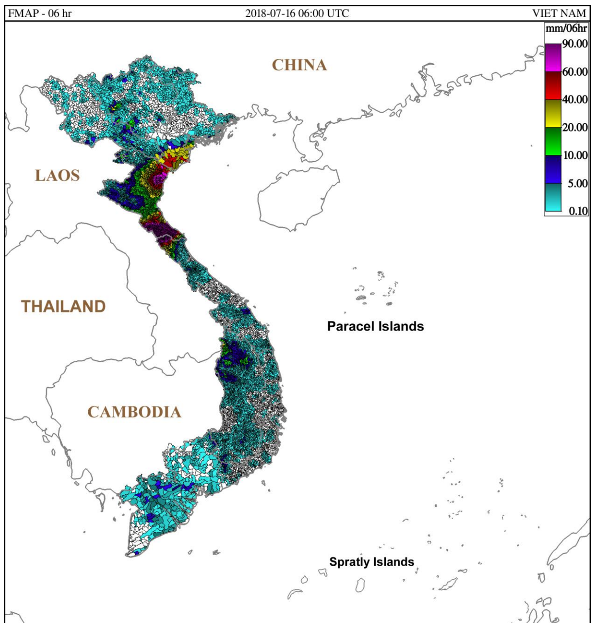
Hình 2: Dự báo lượng mưa trung bình lưu vực 6 giờ tính từ 13h ngày 16/07/2018 giờ địa phương
