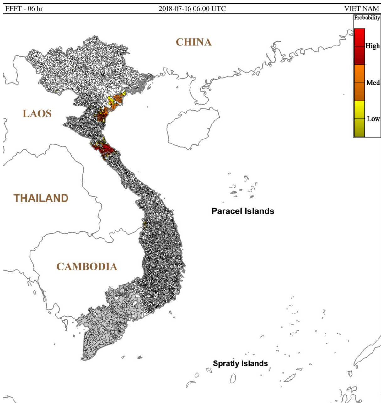
Hình 3: Nguy cơ lũ quét trong 6 giờ tới tại các lưu vực từ 13h ngày 16/07/2018 giờ địa phương
